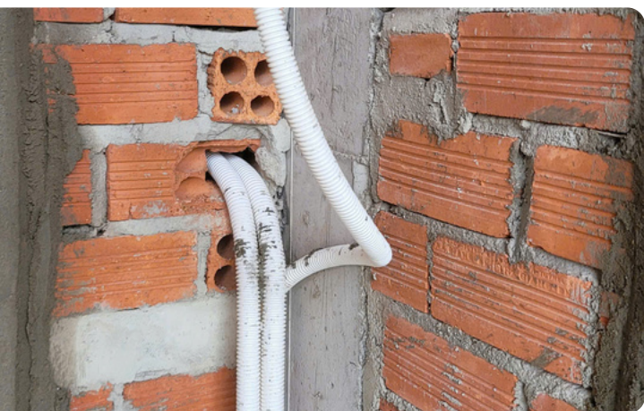
Hình ảnh: Ống đi âm tường
