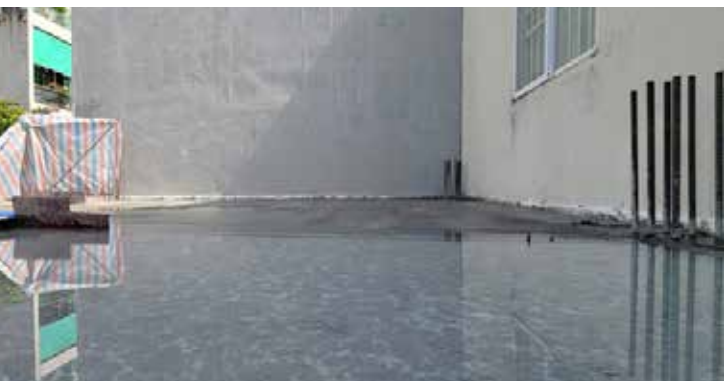
Hình ảnh: Ngâm/tưới bảo dưỡng sau khi đổ bê tông
